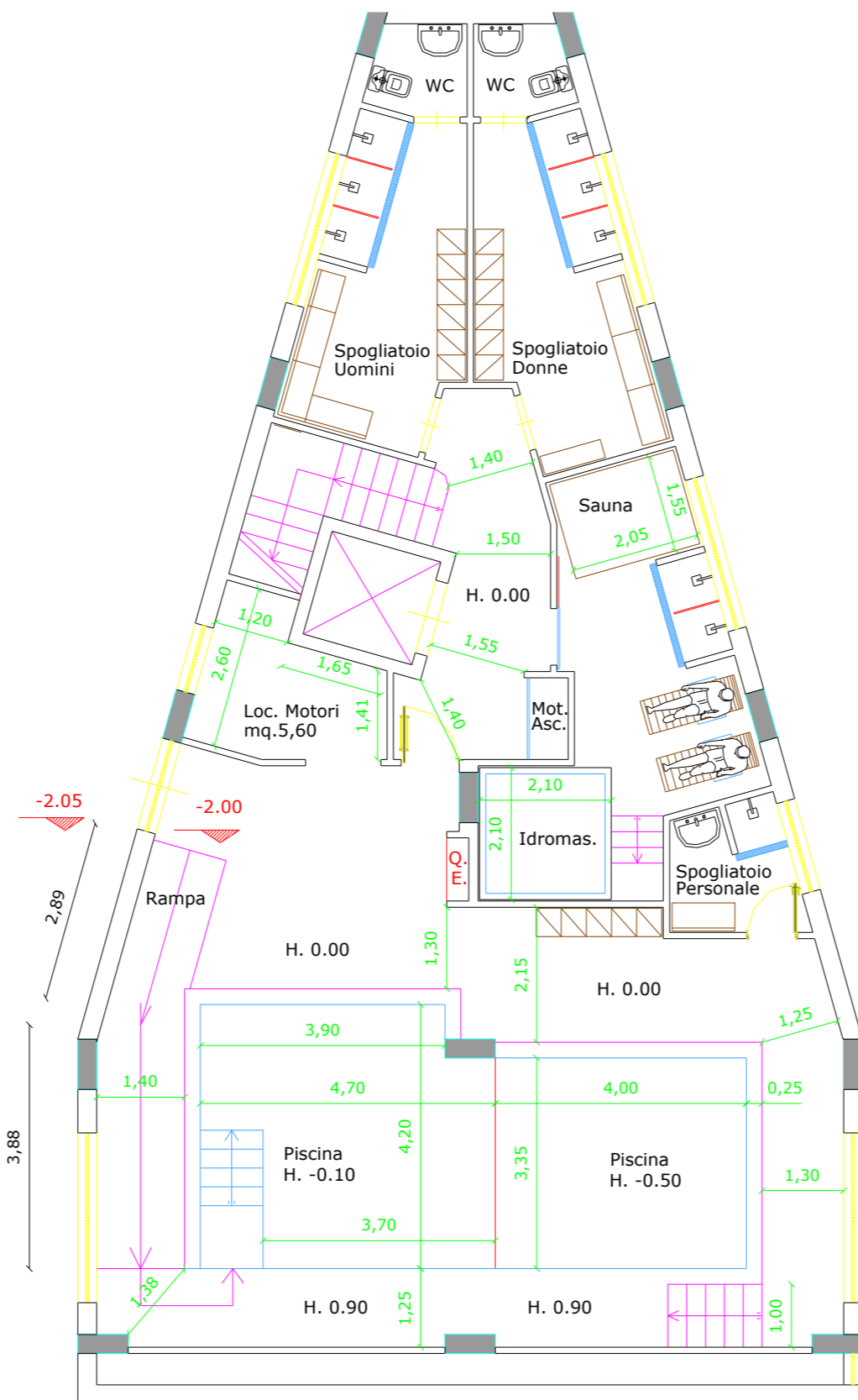
Pianta Piano Cantinato _ scala1:100
